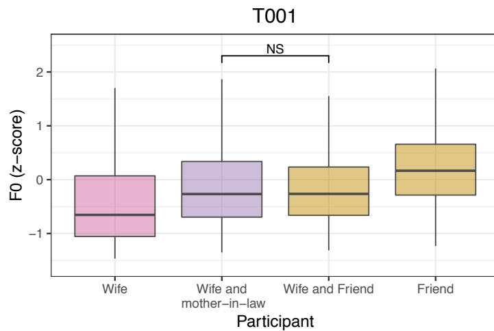
図4 インフォーマント T001 の F0 と会話場面の参加者との関係
