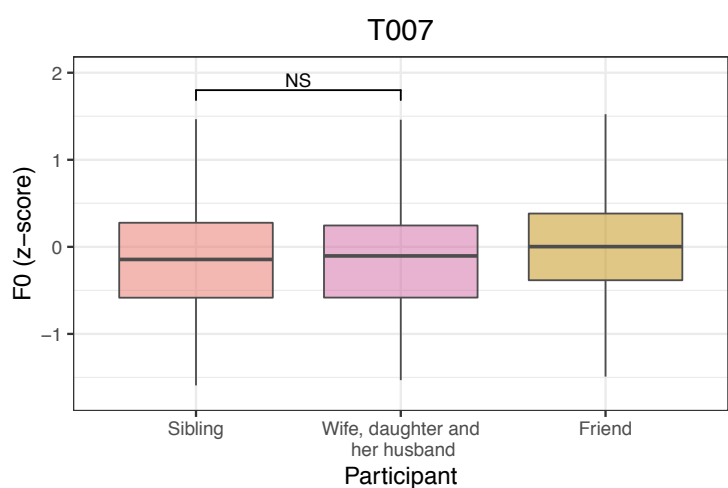
図6 インフォーマント T007 の F0 と会話場面の参与者との関係
