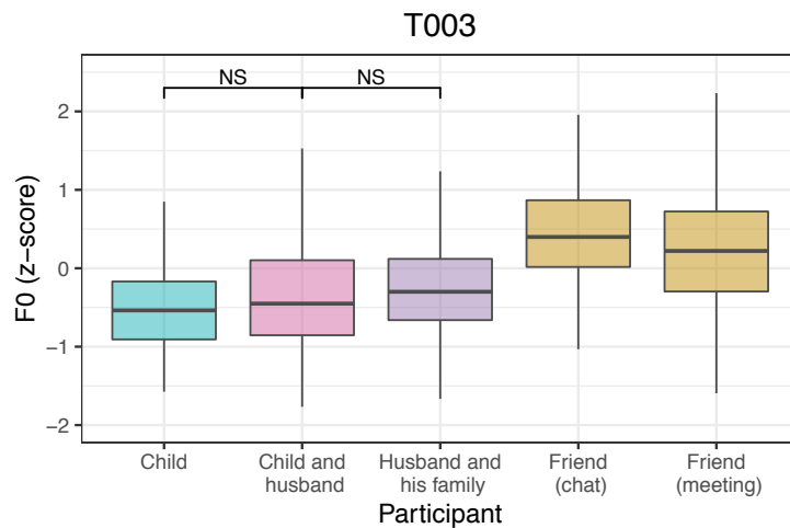
図5 インフォーマント T003 の F0 と会話場面の参加者との関係
