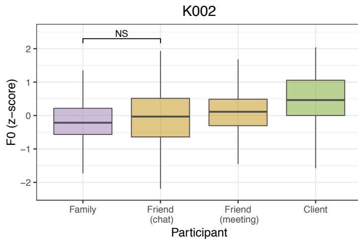
図3 インフォーマント K002 の F0 と会話場面の参加者との関係
