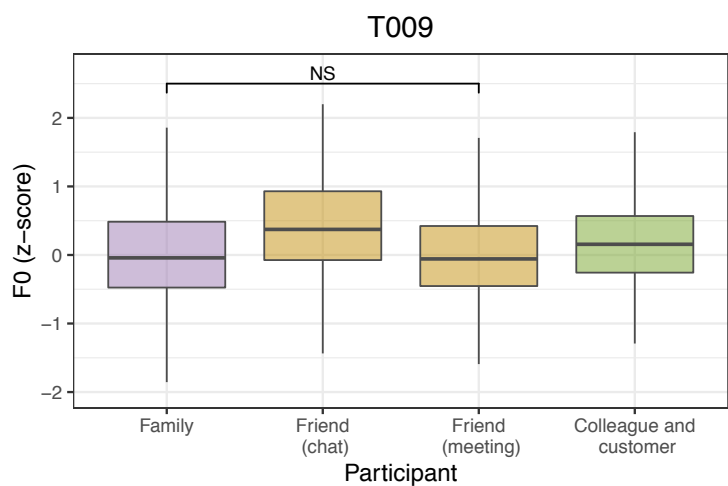
図7 インフォーマント T009 の F0 と会話場面の参与者との関係
