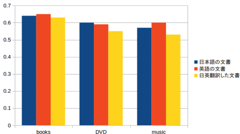
図3 BERT を用いた感情分析
